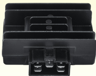
REM2399 Regulador Rectificador 5P Para Yamaha YBR125
