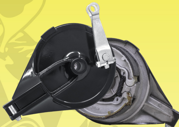
REM2787 Porta balata trasero FORZA - 150 2009-2013, FT 150 GT, FT 150 Grafito
