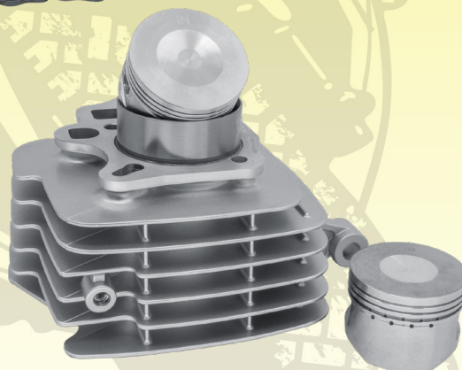
REM145 Cilindro con pistón y anillos Para sport city 110, Metro 110 Dinamo, intrepida 110 Dinamo, Argenta 110
