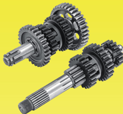
REM3226 Caja de velocidades Engrane primario y secundario para 125FL 19-20
